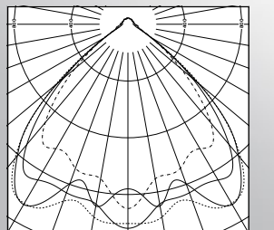
PL33T – für Ausleuchtung von Ecken
