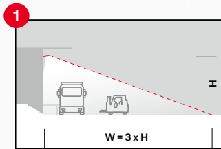
PL43 – für tiefstrahlende Ausleuchtung von Plätzen
