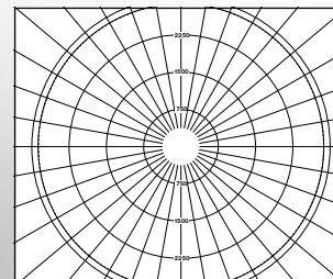
RS07 | RS08 | RS12 – für Mirror- tec-Anwendungen und Hallen
