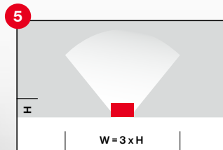
PL33T – für Ausleuchtung von Ecken
