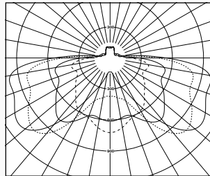
PL52 – für Ausleuchtung von breiten Straßen und Parkplätzen
