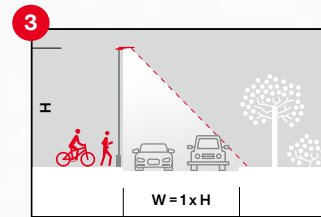
PL61 – für Ausleuchtung von Straßen mit hohen Lichtpunktabständen
