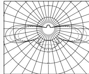
PL61 – für Ausleuchtung von Straßen mit hohen Lichtpunktabständen
