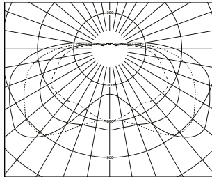
PL43 – für tiefstrahlende Ausleuchtung von Plätzen
