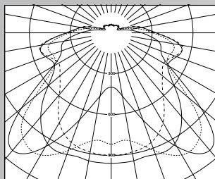
PL64 – für tiefstrahlende Ausleuchtung von Plätzen
